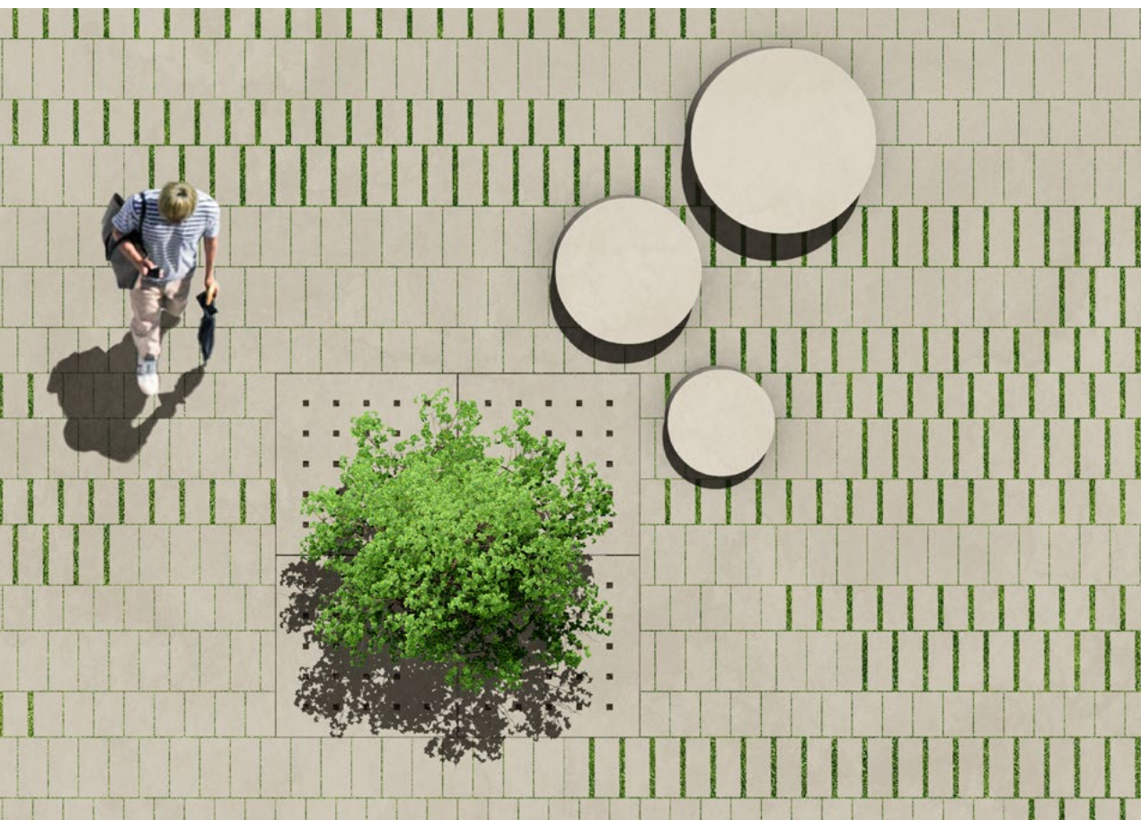
GDM.TETRAGO liner 40/20/8 und 30/20/8 cm mit 30 mm Fuge und GDM.TETRAGO stone 40/20/8 und 30/20/8 cm
